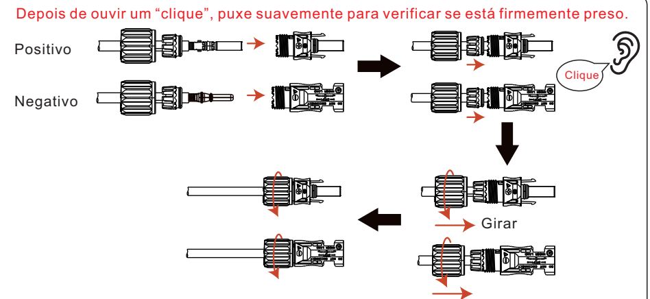
Figura 5.14 Montagem da tampa do conector do terminal
