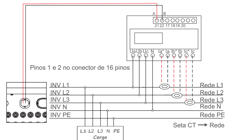
Figura 6.11 Medidor Tipo TC Externo - "Medidor na Rede"
