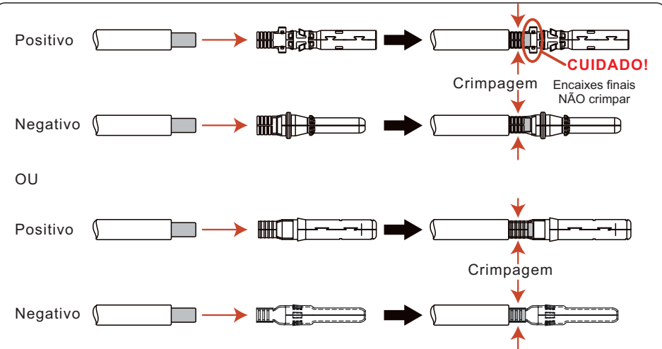
Figura 5.13 Crimpagem
