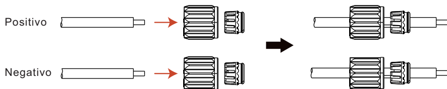
Figura 5.12 Passe o cabo
