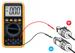
Figura 5.15 Medição com multímetro
