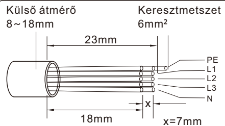
5.20. ábra Lecsupaszított és szabad vezeték
