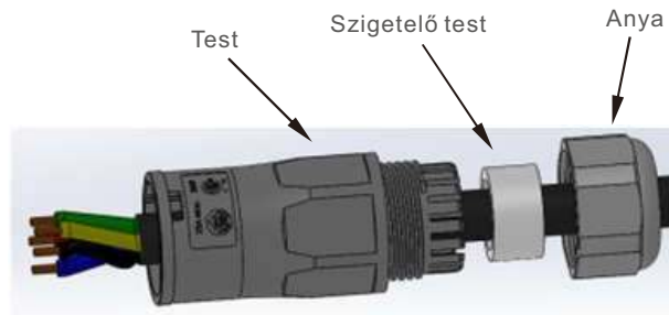
5.19. ábra Váltóáramú csatlakozó
