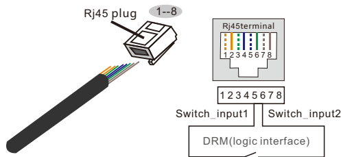
5.31. ábra Csupaszítsa le a szigetelőréteget és csatlakoztassa az RJ45 csatlakozójához
