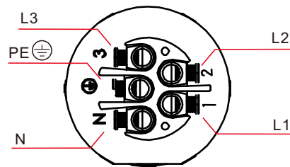
5.21. ábra A váltóáramú csatlakozó belső szerkezete
