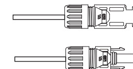
5.16. ábra Csatlakozó rácsavarozott sapkaanyával
