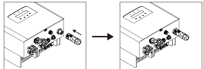
5.24. ábra váltóáramú csatlakozó bekötése az inverterre
