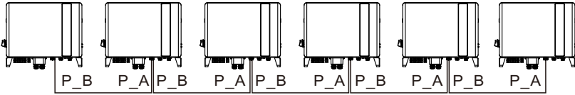
Figura 4.37 Conexión de terminales en paralelo
