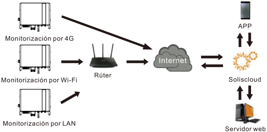
Figura 4.42 Función de comunicación inalámbrica
